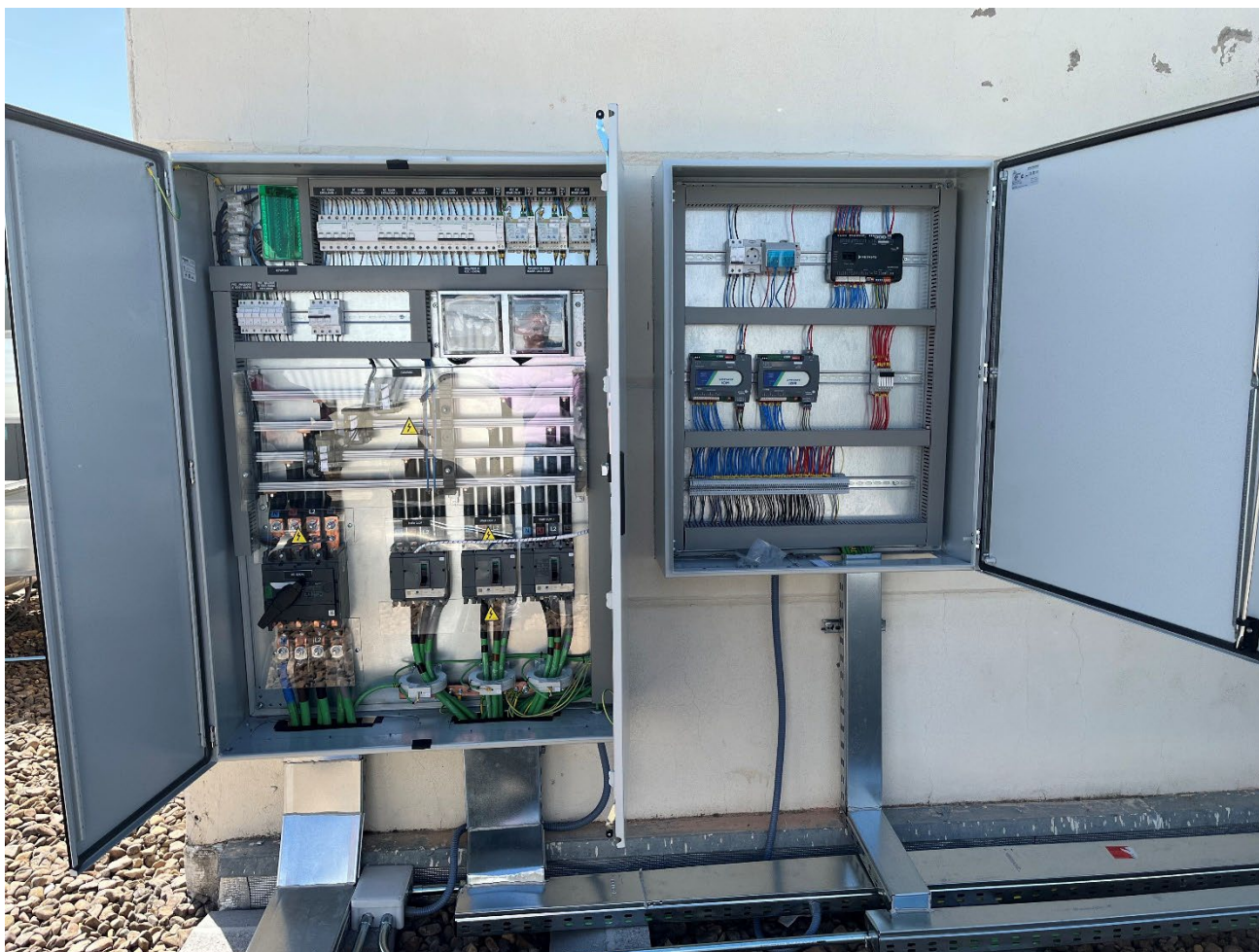
Ilustración 7: Cuadro eléctrico de mando y protección. Cuadro de Control.
